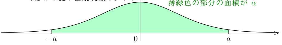
t 分布の確率密度関数のグラフ↑
