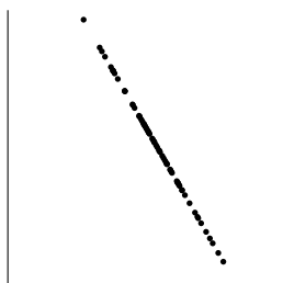
相関係数 -1
