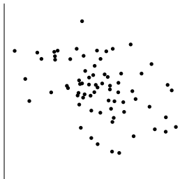
相関係数 -0.4
