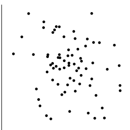
相関係数 -0.2
