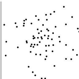
相関係数 0
