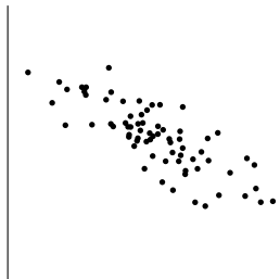
相関係数 -0.8
