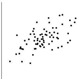
相関係数 0.6
