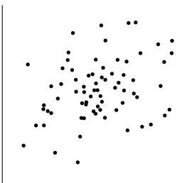
相関係数 0.3
