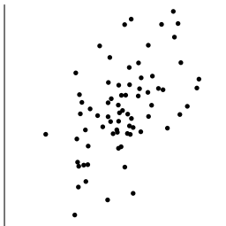
相関係数 0.5
