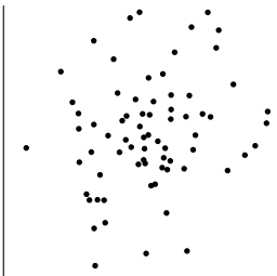
相関係数 0.2
