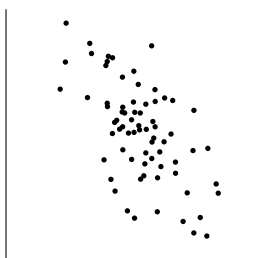
相関係数 -0.6
