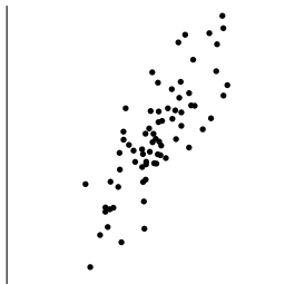
相関係数 0.8
