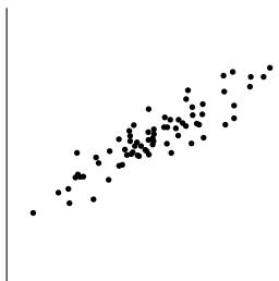
相関係数 0.9
